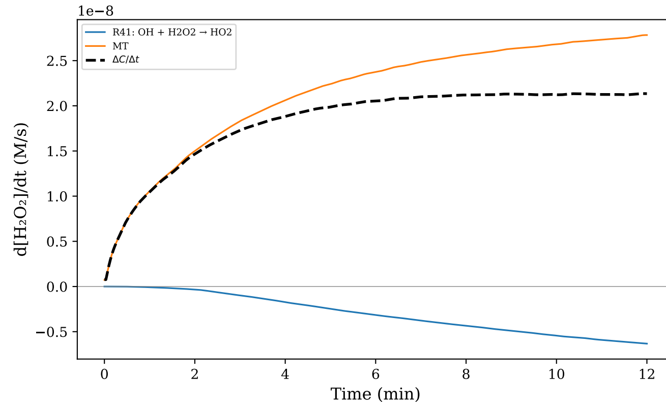
(d) \text{H}_2\text{O}_2
